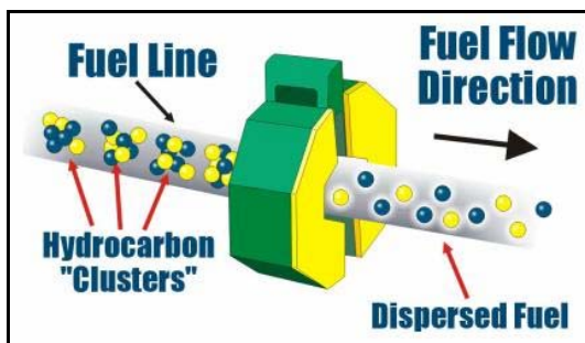
Gambar 3. De-clustering Molekul Hidrokarbon yang Melewati Medan Magnet [10].
