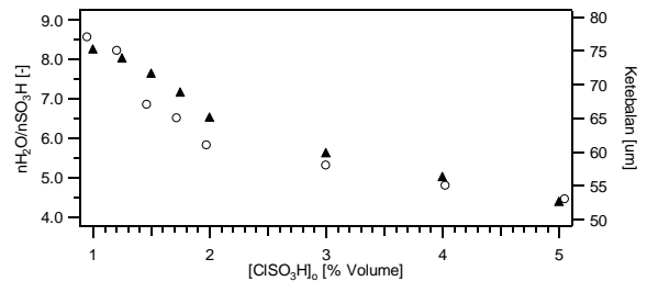
Gambar 4. Pengaruh konsentrasi \text{ClSO}_3\text{H} terhadap \text{KPI}_{\text{membran}} , PA, dan KP. Sulfonasi dilakukan pada suhu kamar selama 8 jam.
